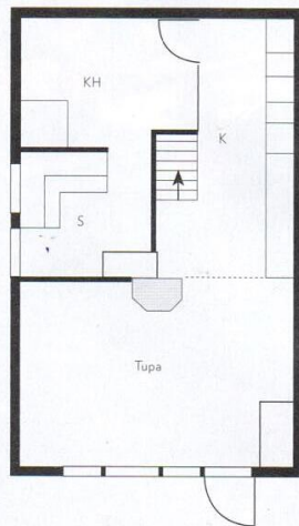
45 neliön mökkiin mahtuvat tupa, keittiönurkka, pesutilat ja sauna.
